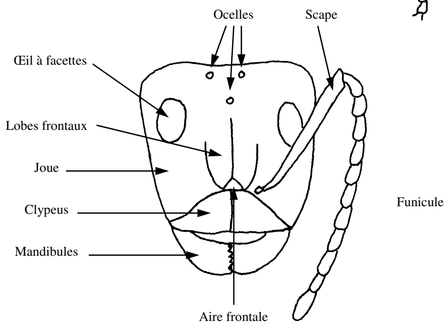
Vue de face d'une tête d'ouvrière du type Formica
